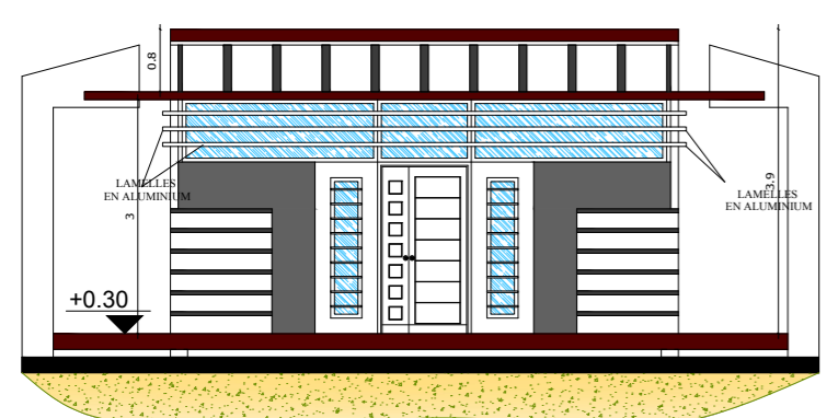
FAÇADE PRINCIPALE ECH 1 / 50
