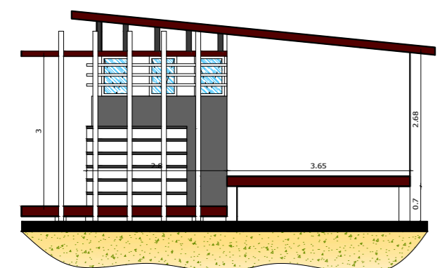
FAÇADE DROITE ET GAUCHE ECH 1 / 50
